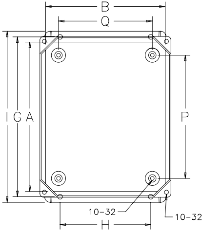
Vista superior sin la puerta y tapa
