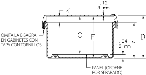
SECCIÓN X-X
